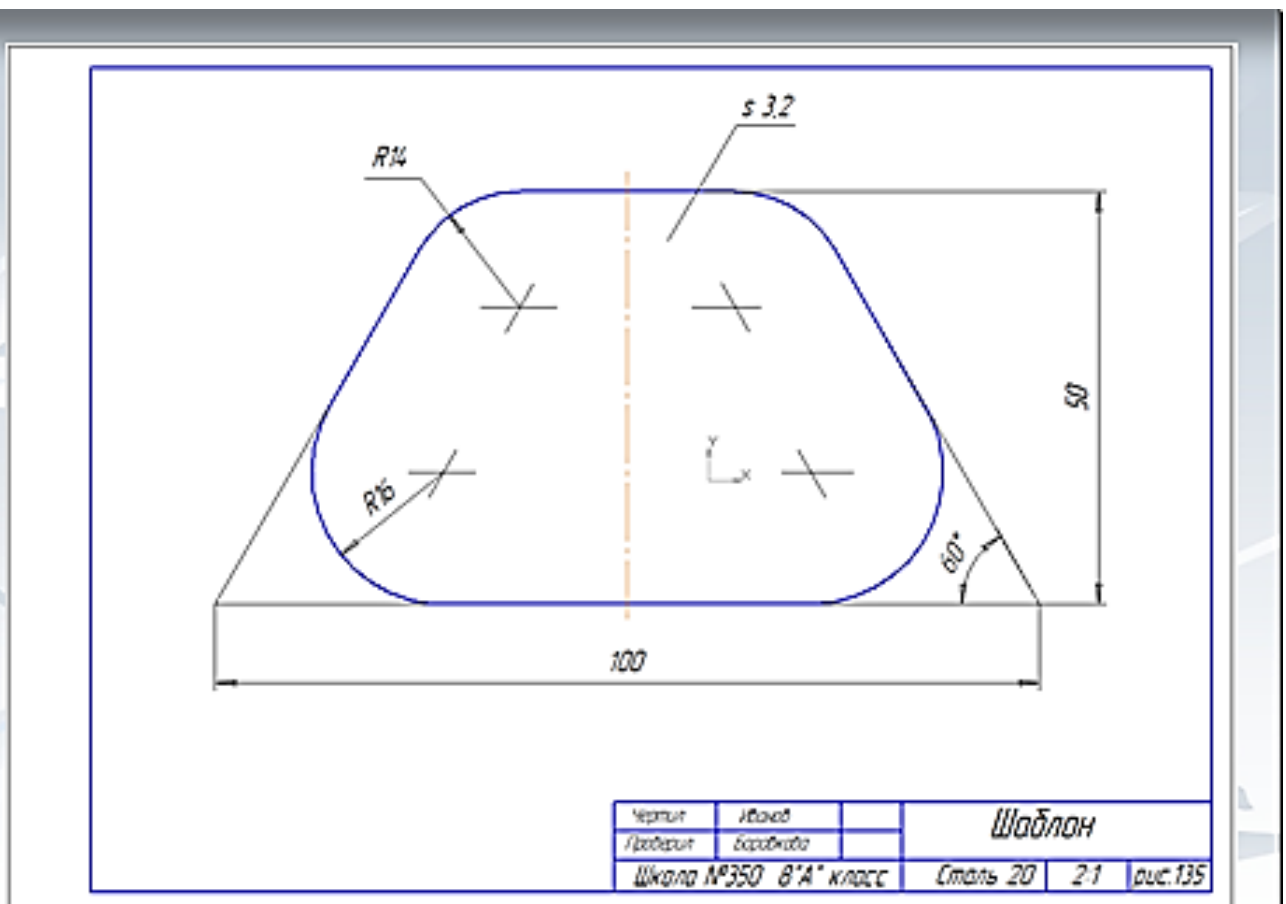
Пример выполнения домашнего задания - чертёж «Шаблон» в М2:1 по рис.135.
